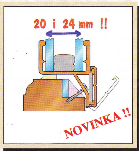
Řez renovovaným zdvojeným oknem
